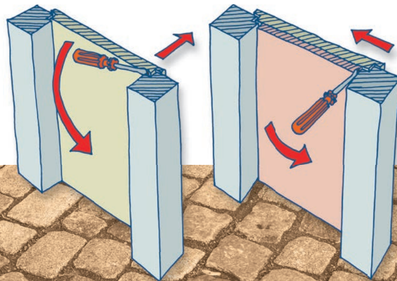
Wenn die Aussenseite einer Tür mit einer zusätzlichen Holzplatte verstärkt wird, kann der Hebel nicht mehr zwischen Tür und Rahmeninnenseite (Zeichnung links) angesetzt werden, sondern nur noch – völlig wirkungslos! – zwischen Rahmen und Holzplatte (Zeichnung rechts).
